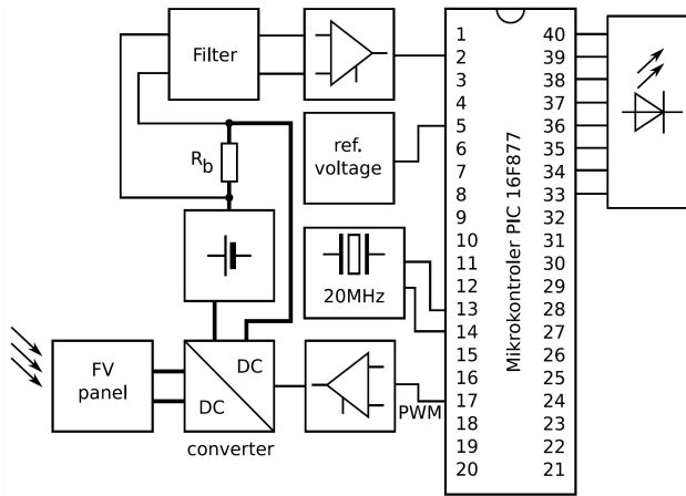
Fig. 27. Optimization circuit.
